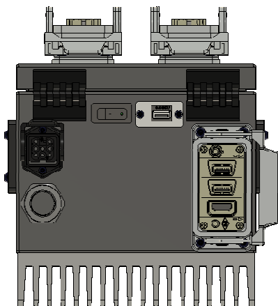
Abb.: Unterseite mit Schnittstellen
